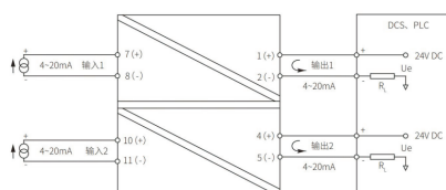
接线图
