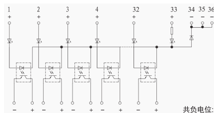
电气原理图
